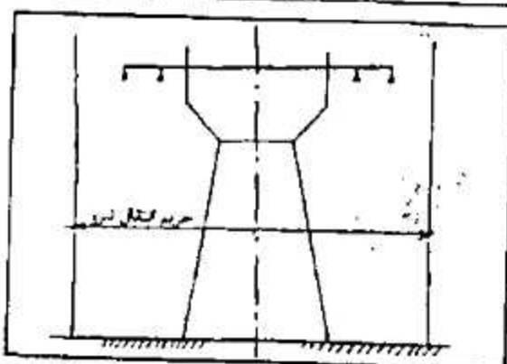
تصویر ۱- حریم انتقال نیروی فشار قوی
