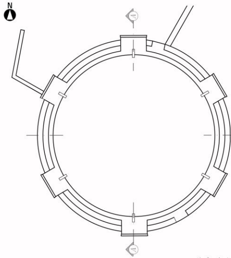
تصویر شماره ۶: پلان
