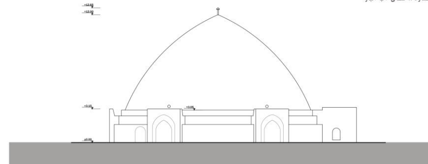
تصویر شماره ۳: نمای آب انبار
