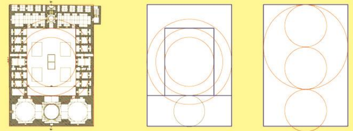
تناسبات هندسی در پلان - مدرسه سردار قزوین
