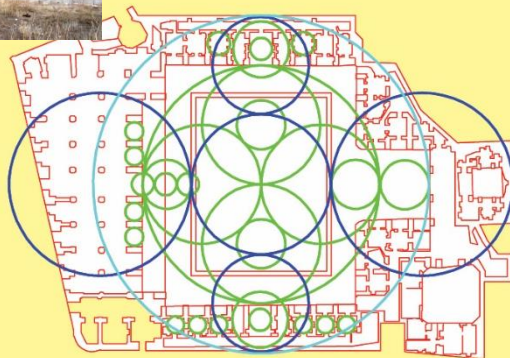
تناسبات هندسی در پلان - مدرسه صالحیه قزوین
